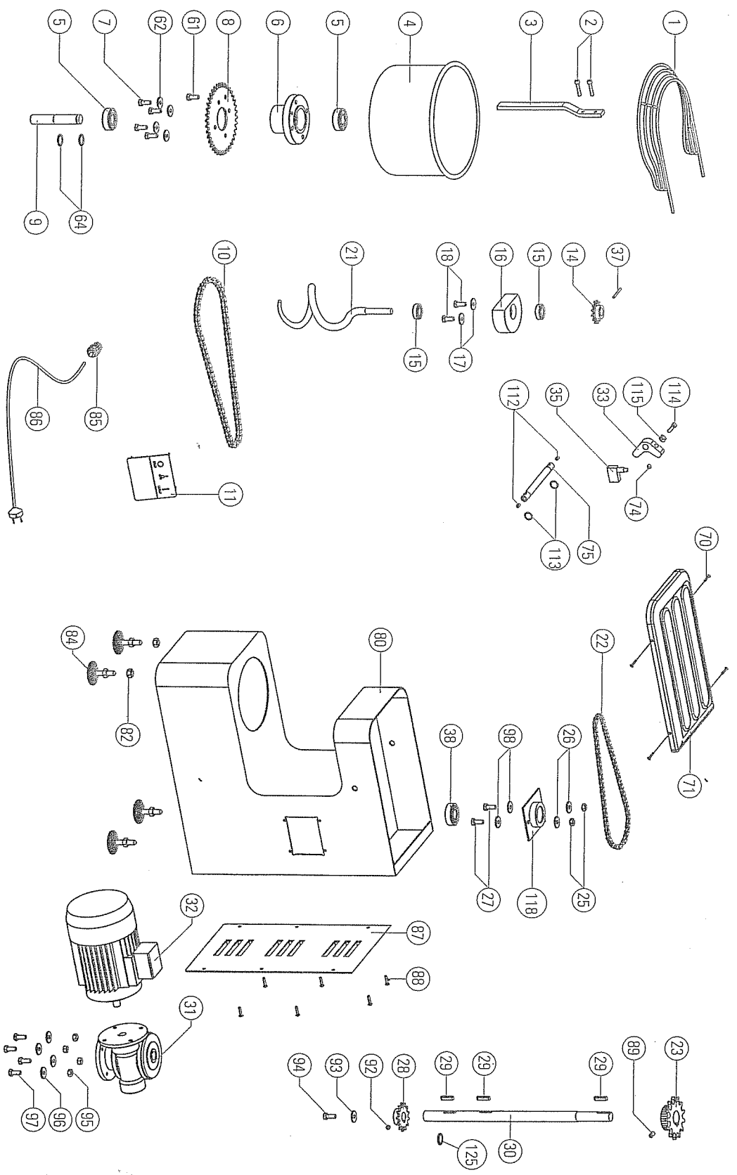
FIG. 17 Pièces de rechange pour pétrisseuse avec tête et cuve fixe mod. PK 5-8 BILD 17 Ersatzteile für die Teigknetmaschine mit gestem Kopf und Becken mod. PK 5-8
