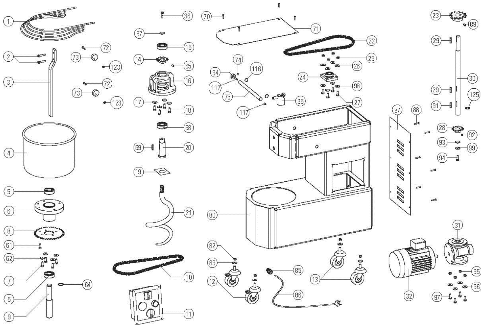
BILD 19 Ersatzteile für die Teigknetmaschine mit gestem Kopf und Becken mod. IM 25-38-44
