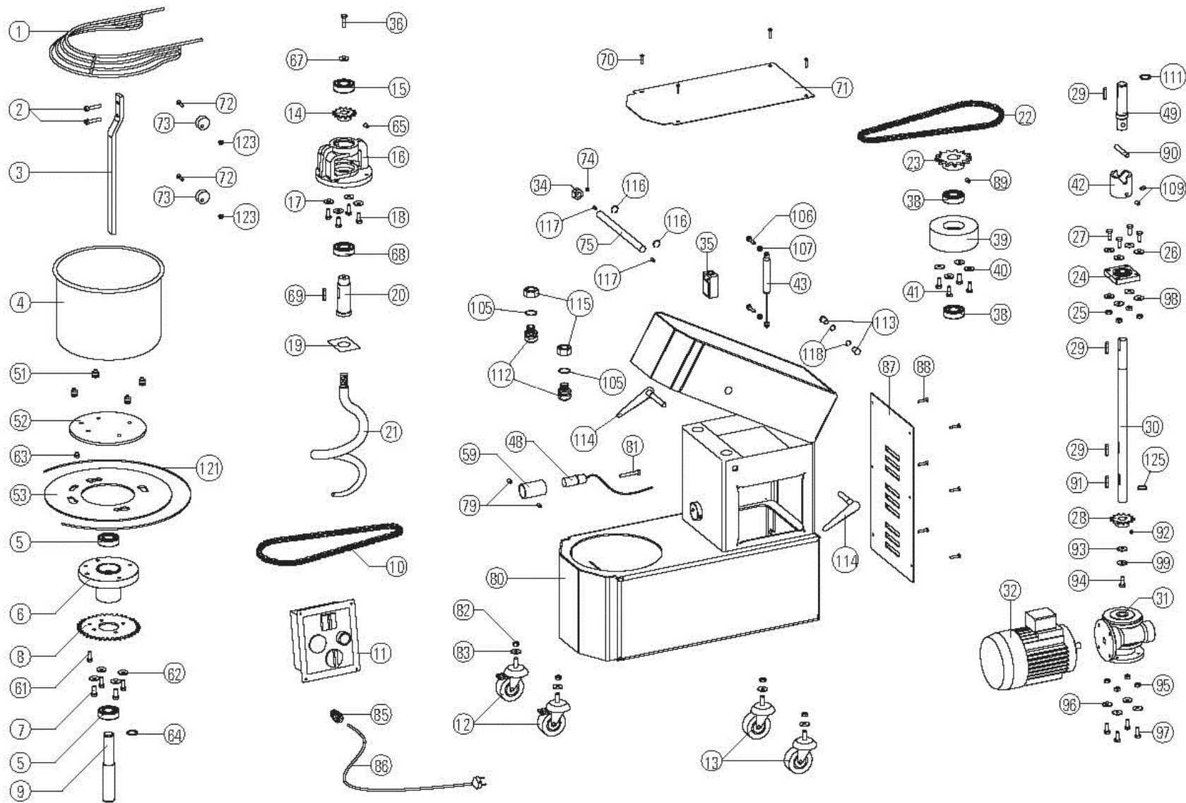
FIG. 22 Parti di ricambio impastatrice con testa sollevabile e vasca estraibile mod. IM 25-38-44 A PICT. 22 Spare parts for mixer with raising top and removable bowl mod. IM 25-38-44 A
