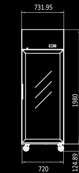
MCF8604 MCF8601
